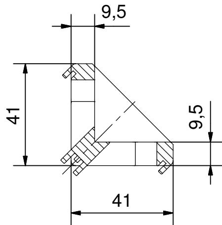
Aluminiumdruckguß
